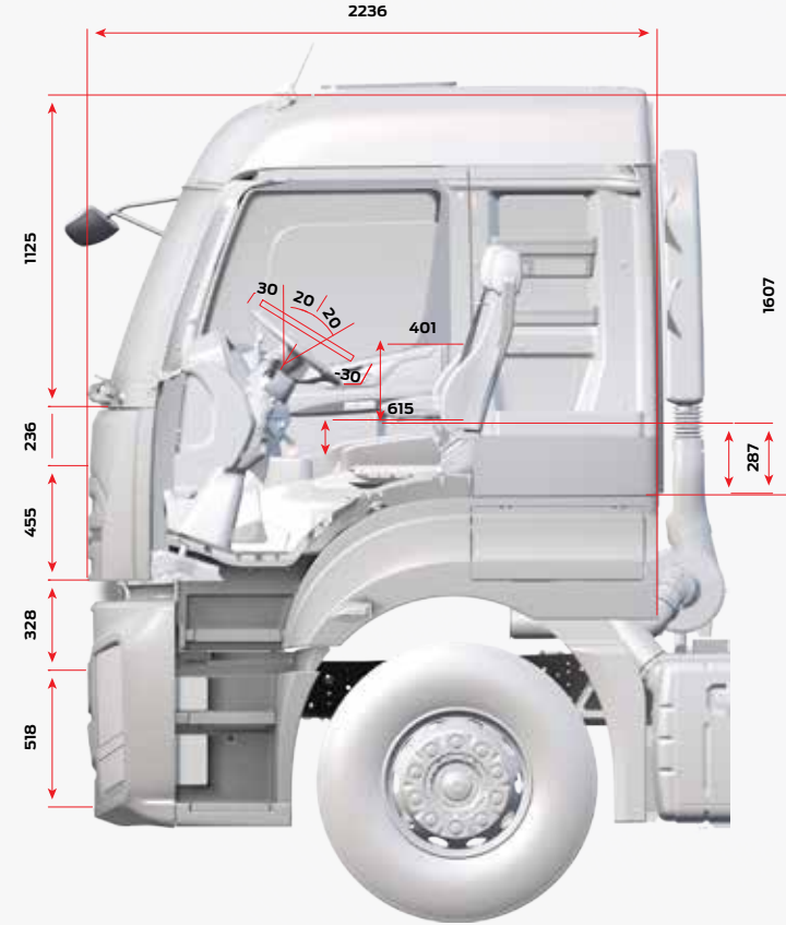
YÜKSEK TAVAN YATAKLI KABİN
