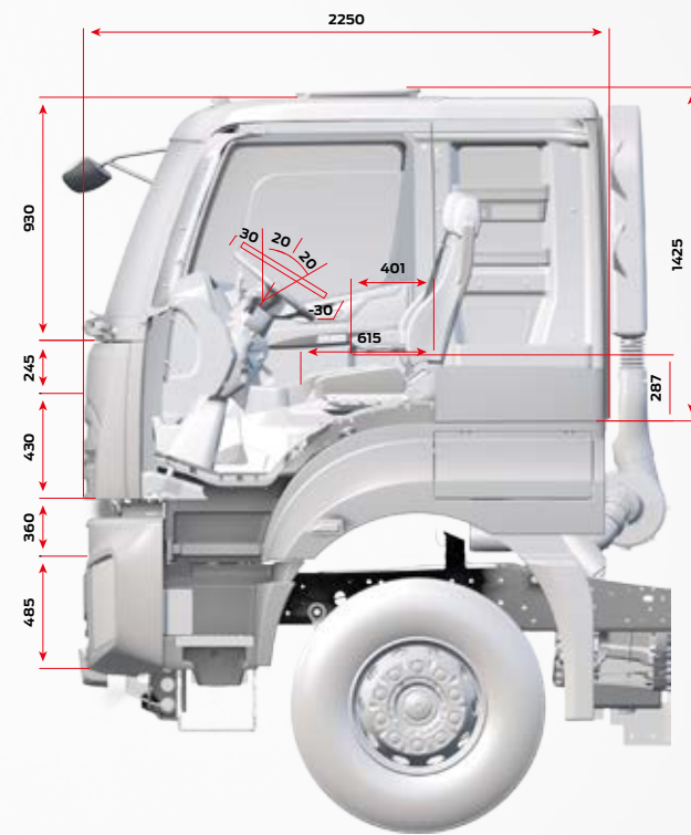
CABINE COUCHETTE À TOIT SURBAISSÉ
