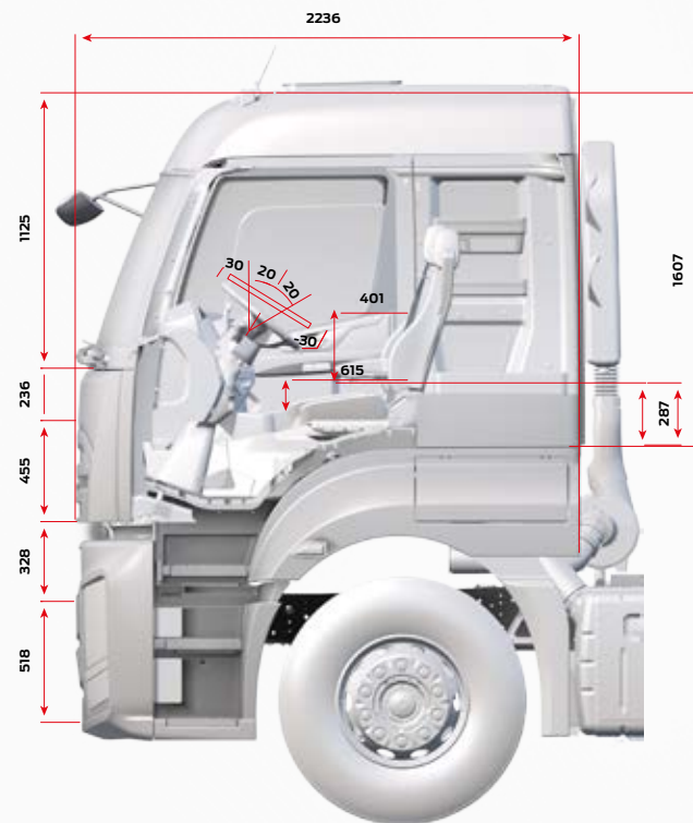
CABINE COUCHETTE À TOIT SURÉLEVÉ
