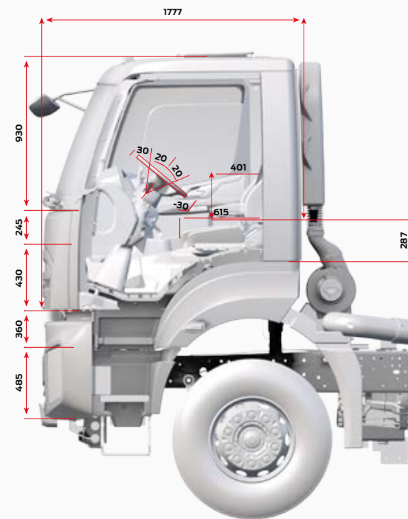
CABINE DE JOUR À TOIT SURBAISSÉ
