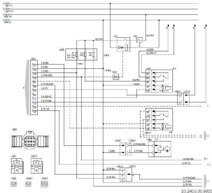
Kablo ağacı devre planı 12 Volt / 24 Volt / ADR
