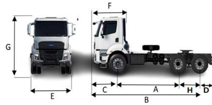
3551T Yataksız Kabin
